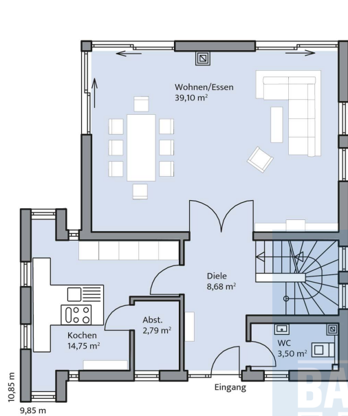
Haus Haas Grundriss
